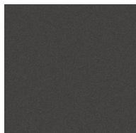
Arena de peltre
